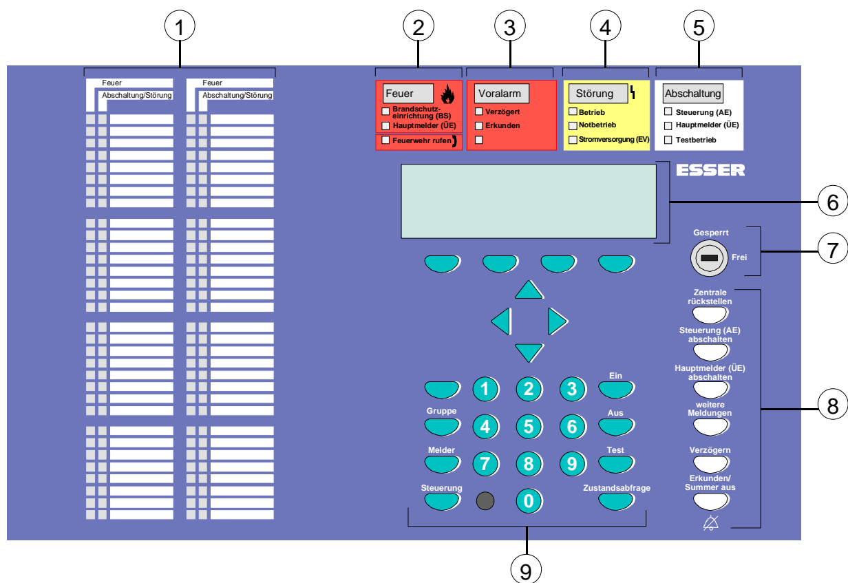
Obr. 1 Celkový pohled na signalizační a ovládací prvky
